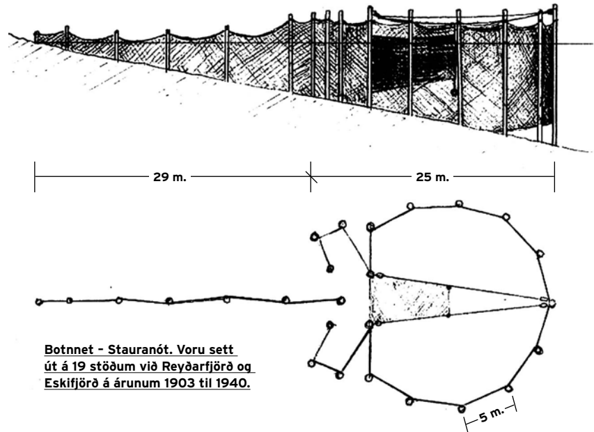
Teikning af stauranót eftir Geir Hólm frá 2019.
