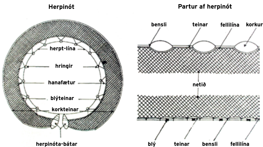
Uppdráttur, er sýnir aðalfyrirkomulag herpinótar.
