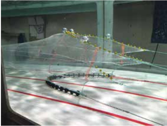
Verið að prófa botntroll í veiðarfæratanki.
